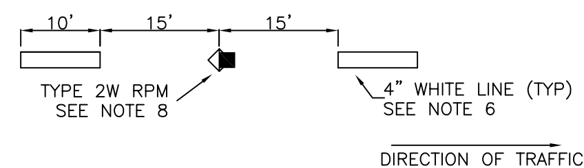
LANE LINE (LL)
