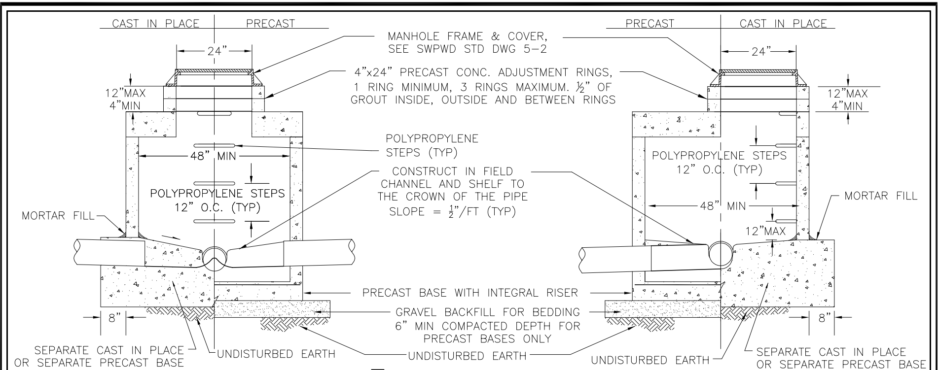
SECTION A-A
